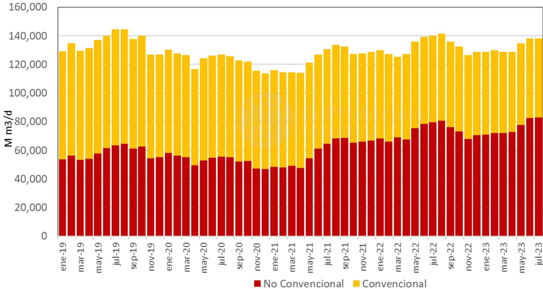
Producción de Gas Convencional y No Convencional - JULIO 2023
