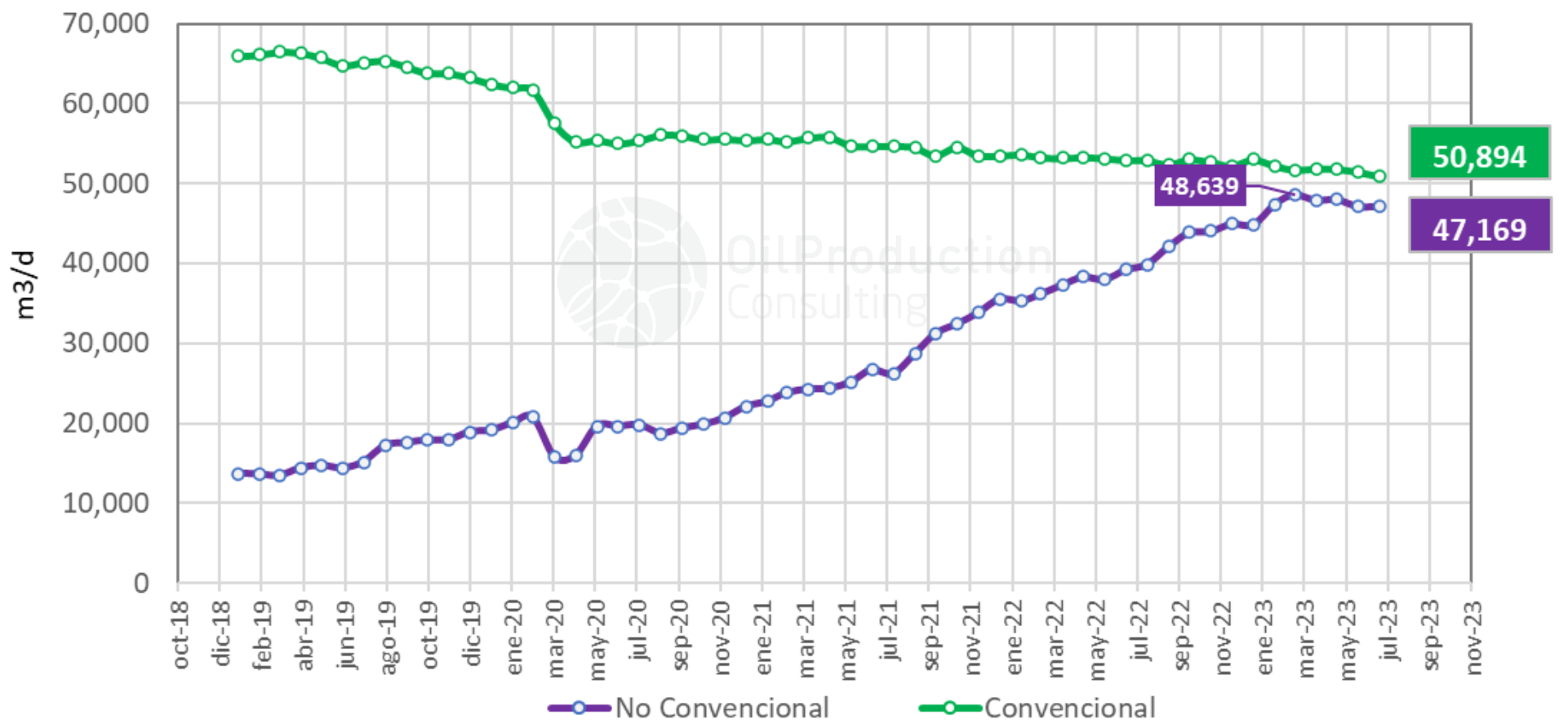
PRODUCCIÓN DE PETRÓLEO CONVENCIONAL Y NO CONVENCIONAL - JULIO 2023
